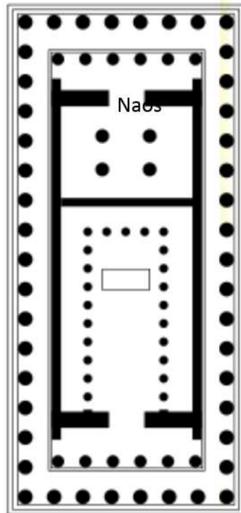
Plan du temple grecque Parthénon d'Athènes
